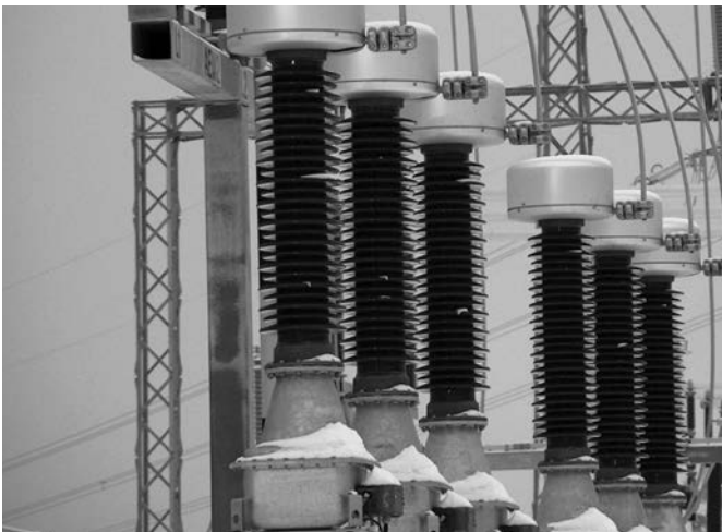
UT 123 ÷ 245 kV
